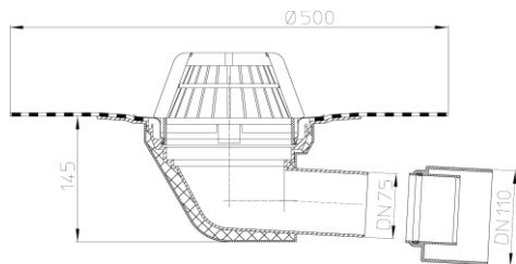
Рис. 1. Кровельная воронка HL64H.
