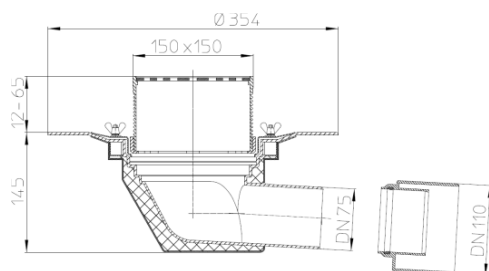
Рис. 1. Кровельная воронка HL64B.
