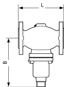
VFG2 (21), VFGS2 D_y 15–125
