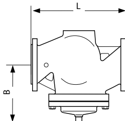
VFG2 (21), VFGS2 D_y 150–250
