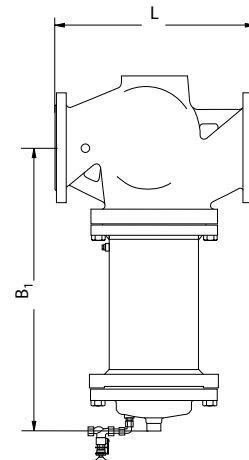
VFG2, VFGS2 D_y 150–250, с удлиненным штоком для T > 140^\circ\text{C}
