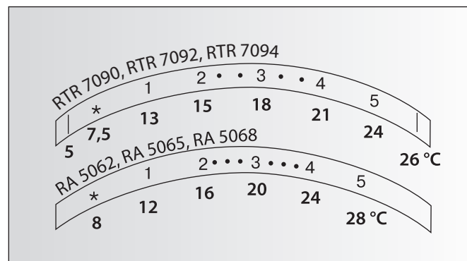
Рис. 4. Шкалы температурной настройки термоэлементов типа RTR.
