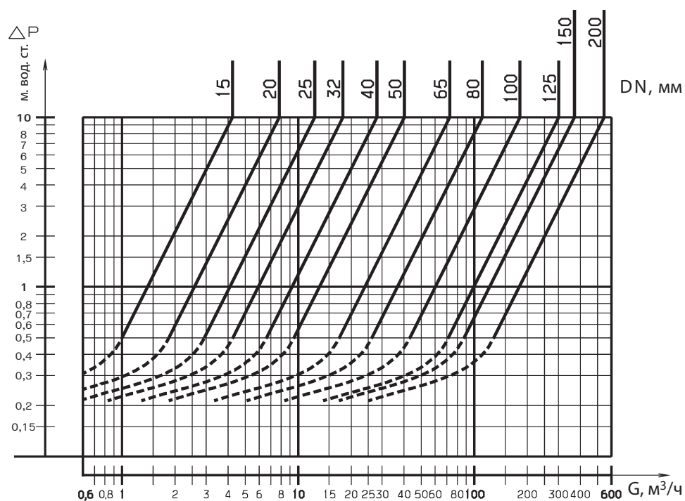
Номограмма потерь давления в клапанах тип NVD 802, NVD 812
